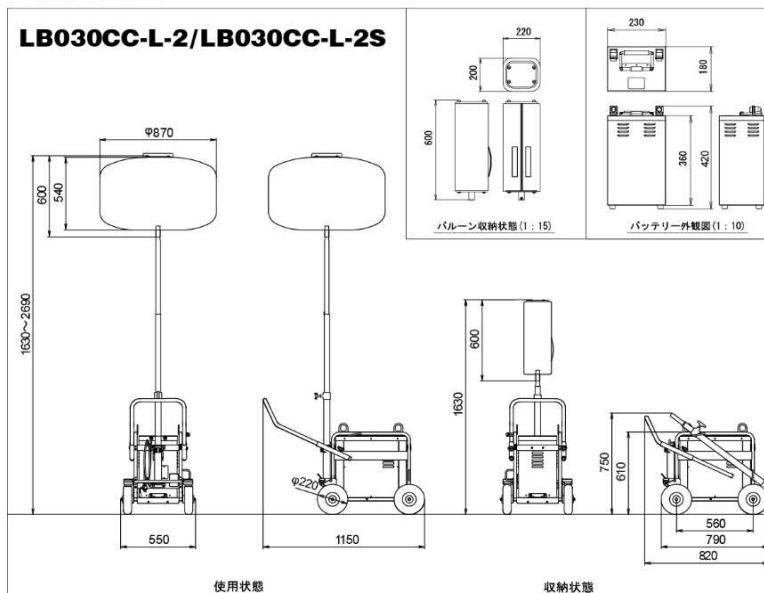
■外形寸法図
